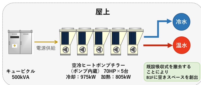
▲熱源システムイメージ
